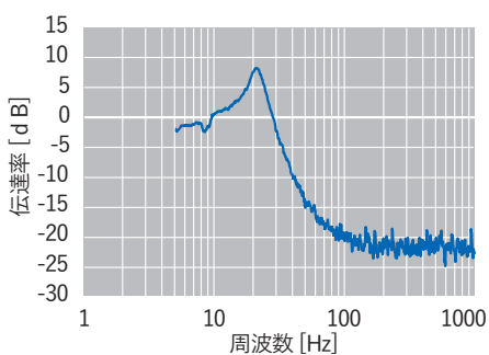
■ 周波数特性
